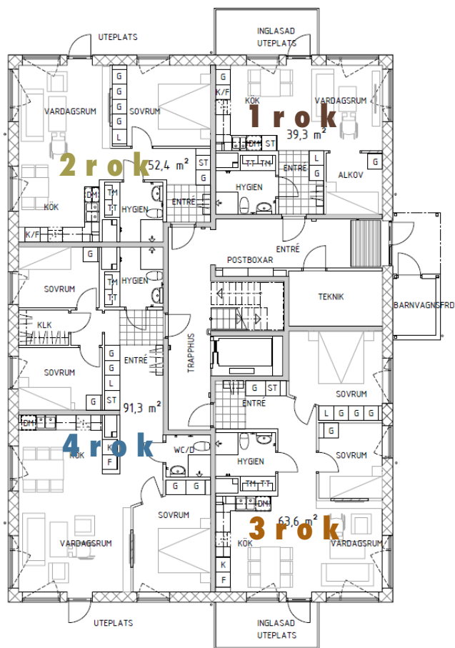
Entréplan
