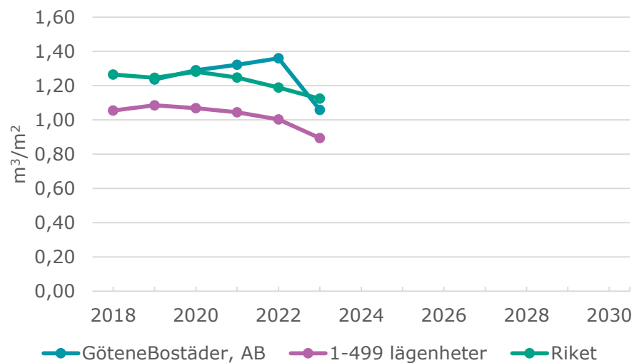
Diagram 3.2.1 Kallvattenanvändning
