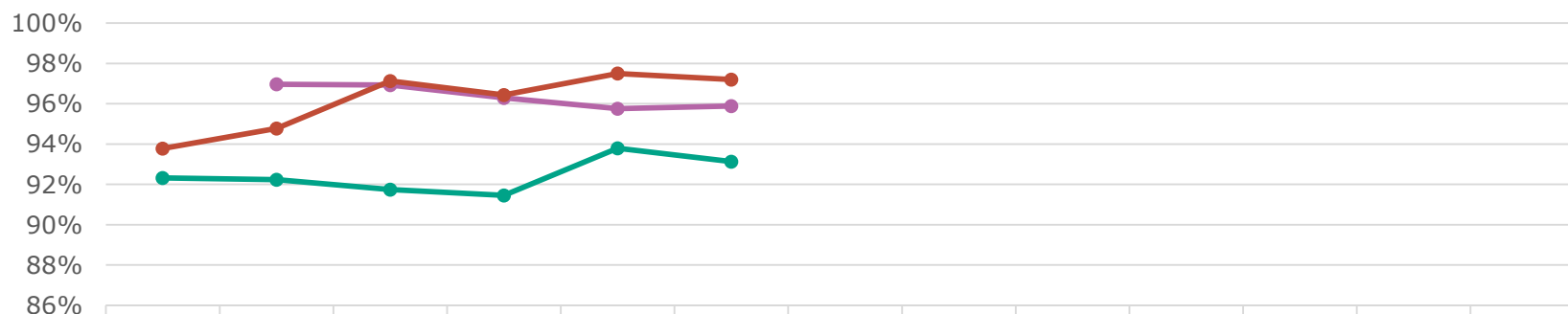
Diagram 1.1 Mål fossilfritt
