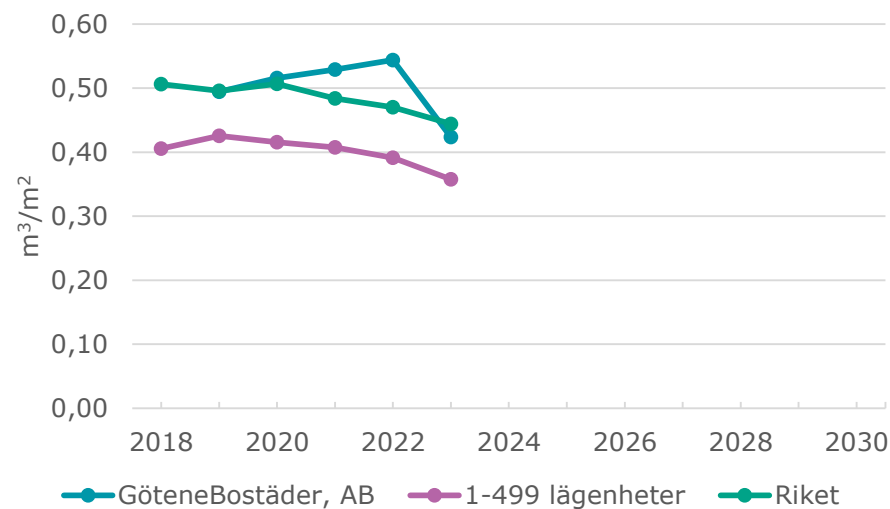
Diagram 3.2.2 Varmvattenanvändning
